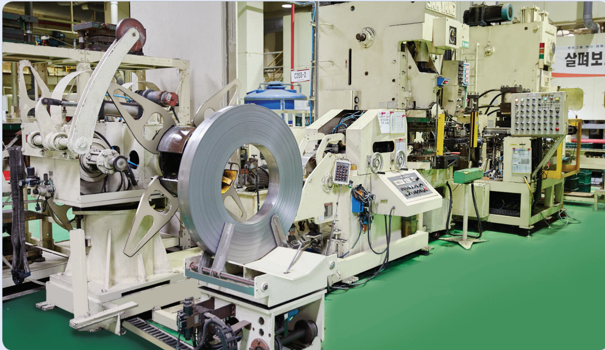
롤 & 싸이징기 / Roll & sizing machine / 롤& 사이징기機
