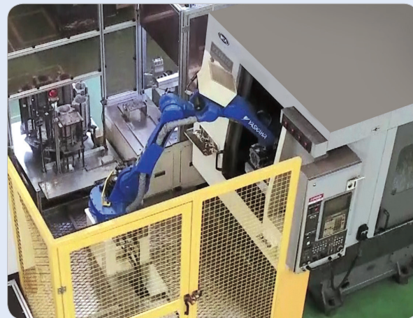
가공 자동화 라인2 / Auto machining line 2 / 自動化 切削加工 라인 2
